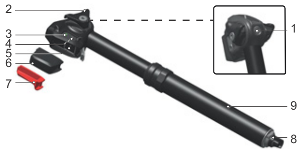
Afbeelding 32: Opbouw ROCKSHOX Reverb AXS verende zadelpen
