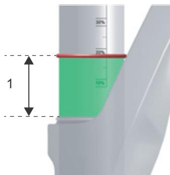
Afbeelding 109: Sag (1)
