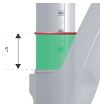
Afbeelding 106: Sag (1)
