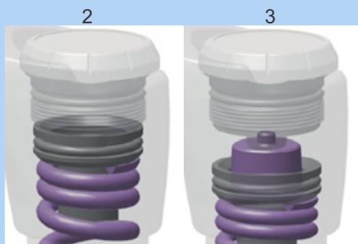
Afbeelding 103: Voorspanningsafstelling in- en uitdraaien
