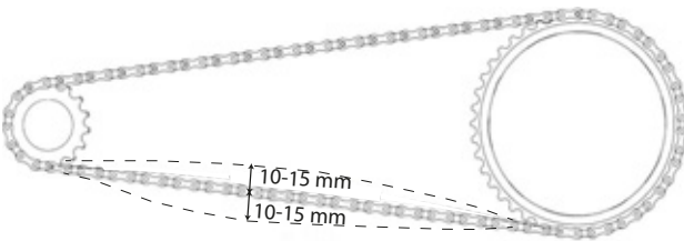
Afbeelding 158: Kettingspanning controleren
