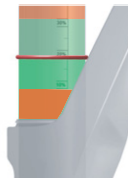
Afbeelding 107: Voorgeschreven sagbereik (groen) en verboden sagbereik (rood)
