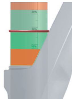
Afbeelding 110: Voorgeschreven sagbereik (groen) en verboden sagbereik (rood)
