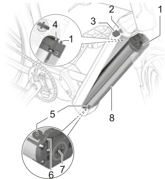
Afbeelding 39: Details PowerTube 750
