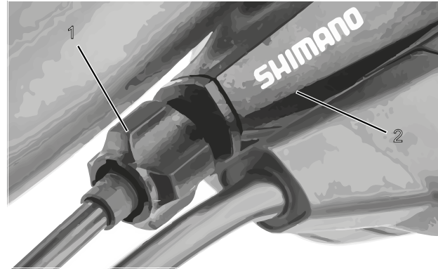
Afbeelding 161: Afstelwartel (1) van de versnelling met enkele bowdenkabelbediening en behuizing van de schakelhendel (2), voorbeeld
