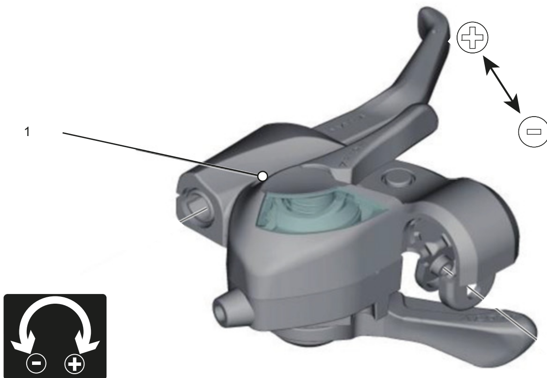
Afbeelding 96: Locatie stelschroef (1)
