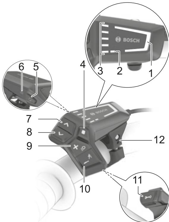
Afbeelding 137: Overzicht bediening BOSCH LED Remote
