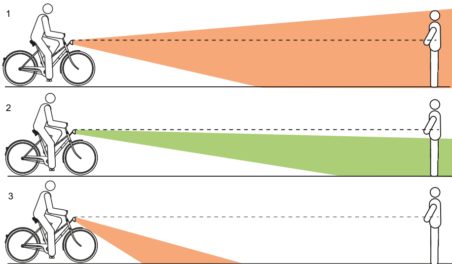
85. ábra: Túl magasra (1), helyesen (2) és túl mélyre (3) beállított világítás
