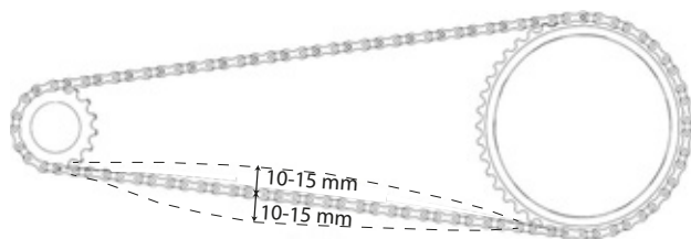
121. ábra: Láncfeszítés ellenőrzése
