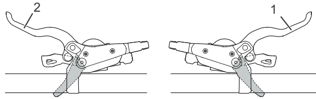
105. ábra: Hátsó (1) és első (2) fékkar, példa: SHIMANO fék
