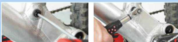
160. ábra: Postpin tengely rögzítése
