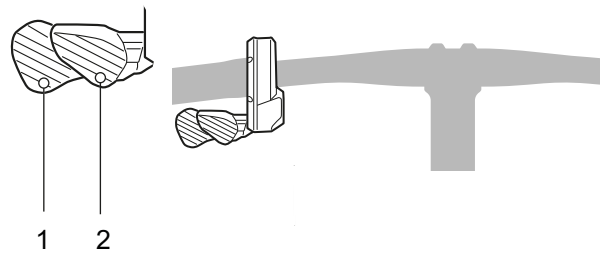
43. ábra: MTB típusú kezelőegység
