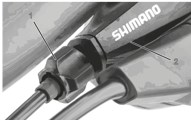
124. ábra: Az egybovdenes, bovdenel működő sebességváltó beállítóhüvelye (1) váltókarházzal (2), példa
