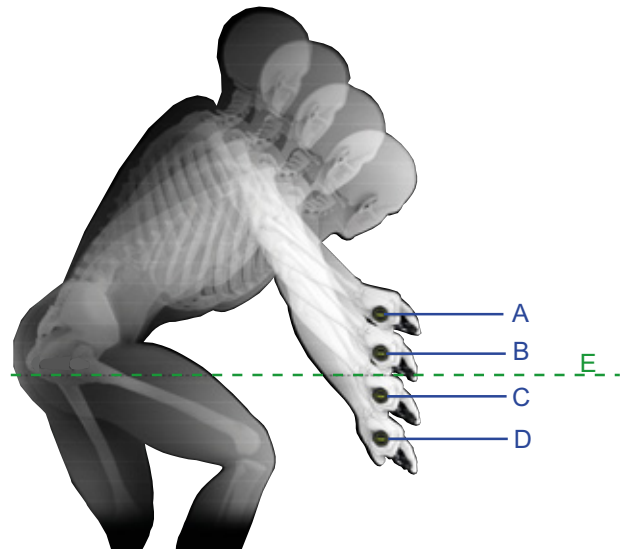
77. ábra: Példa: 4 különböző kormánymagasság (A, B, C és D) és a nyeregmagasság (E)
