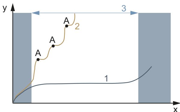
113. ábra: Kopás, üzemidő (x) az anyagledörzsölődés (y) arányában diagram
