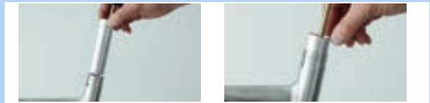
Abbildung 180: Gleitbuchsenrohr ins Sattelrohr stecken
