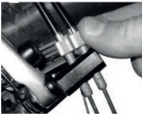
Abbildung 142: ROHLOFF-Naben Versionen mit interner Schaltansteuerung haben die Zugeinsteller am Zuggegenhalter
