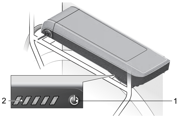
Abbildung 42: Lage Ladezustandsanzeige Gepäckträgerakku
