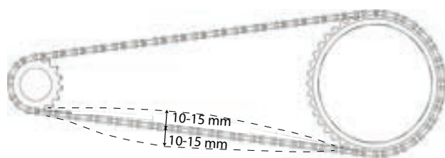
Abbildung 141: Kettenspannung prüfen
