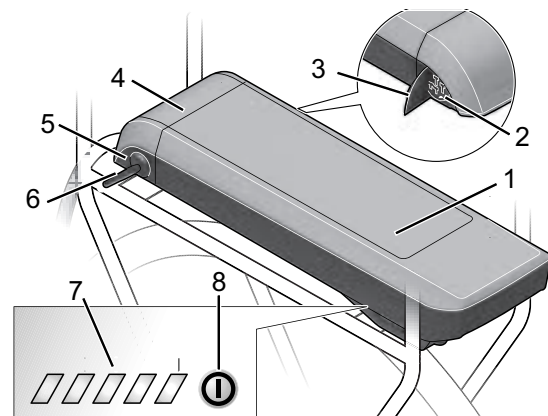
Abbildung 32: Detail Gepäckträgerakku
