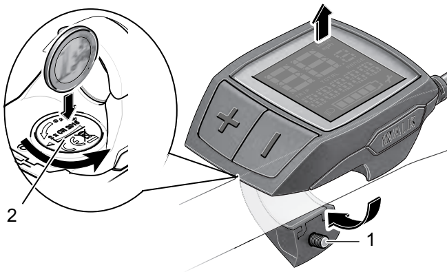
Abbildung 124: Bordcomputer mit Befestigungsschraube (1) und Batteriefachdeckel (2)
