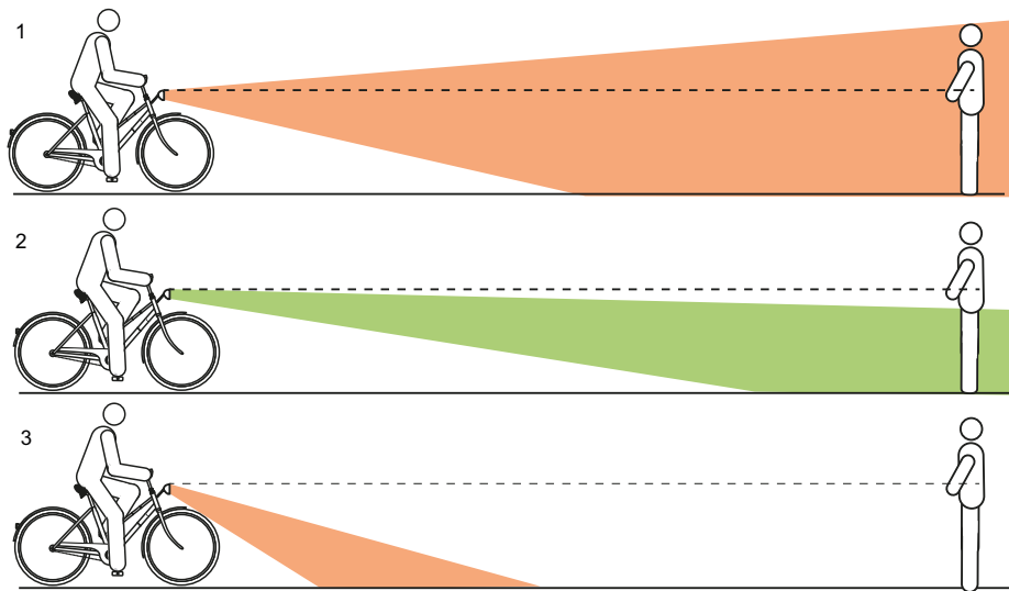
Figura 99: Luz ajustada demasiado alta (1), correctamente (2) y demasiado baja (3)
