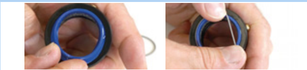
Figura 159: Inserción y fijación del rascador
