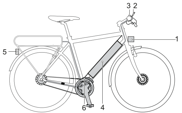
Figura 34: Esquema del sistema de accionamiento eléctrico
