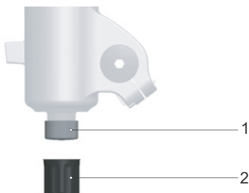
Figura 218: Tornillo de niveles de tracción FOX (1) debajo del capuchón de la horquilla (2)
