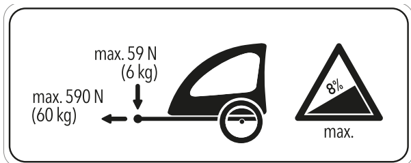
Figura 107: Placa indicadora de remolque
