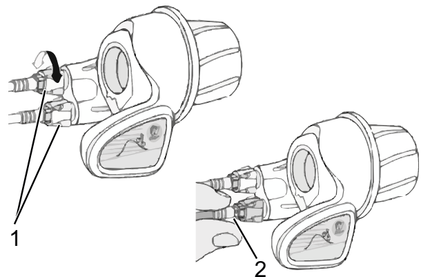
Figura 141: Puño giratorio con casquillos de ajuste (1) y holgura del cambio de marchas (2)
