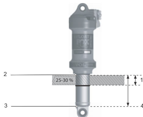
Figura 98: (1) SAG, junta de goma de la cámara de aire (2), junta tórica y recorrido de muelle total del amortiguador
