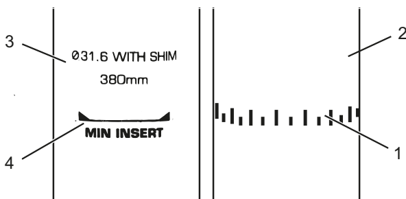
Figura 70: Vista detallada de las tijas de sillín, ejemplos de las marcas de la profundidad de inserción mínima
