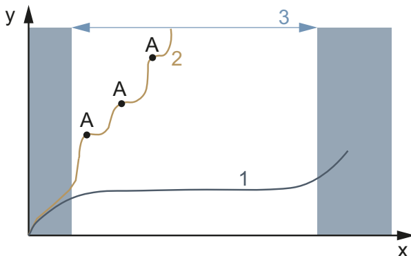
Figura 128: Diagrama de desgaste, vida útil (x) con respecto a desgaste de materiales (y)
