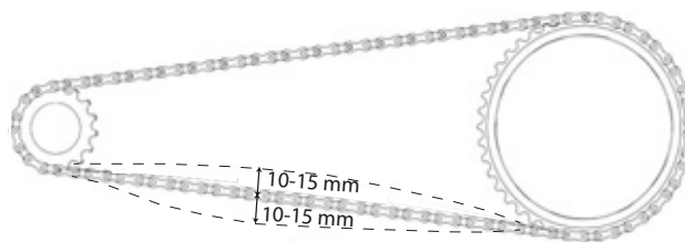
Figura 138: Comprobación de la tensión de la cadena
