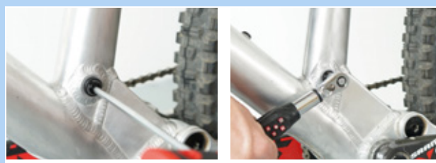
Figura 208: Atornillar la tija de sillín
