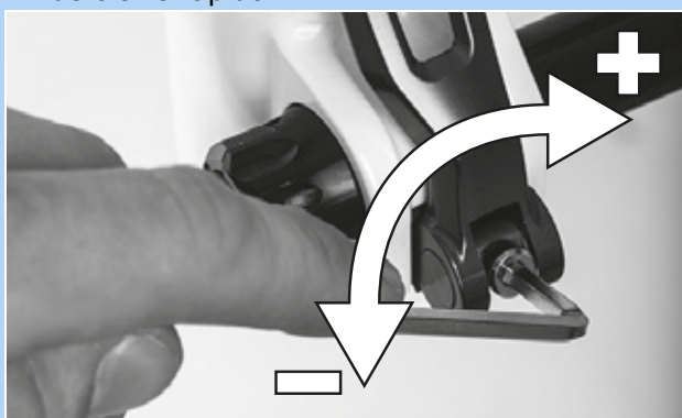
Figura 145: Ajuste de la fuerza de tensado del cierre rápido
