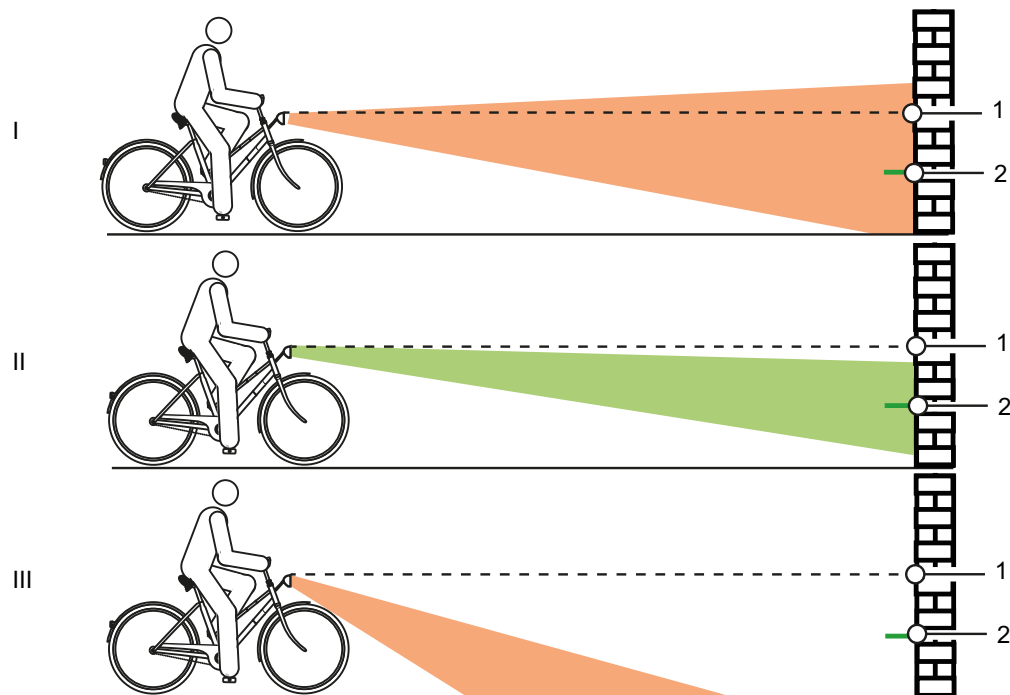
Figura 137: Luz ajustada demasiado alta (1), correctamente (2) y demasiado baja (3)
