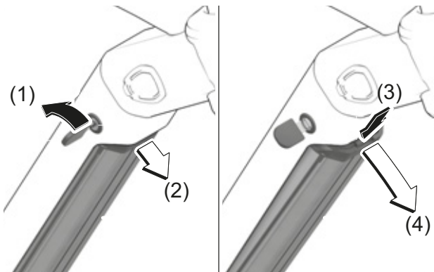
Figura 117: Extracción de la batería
