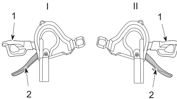
Figura 125: Palanca de cambio hacia abajo (1) y palanca de cambio hacia arriba (2) del cambio de marchas izquierdo (I) y derecho (II)
