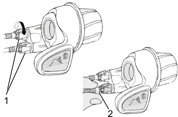
Figura 143: Puño giratorio con casquillos de ajuste (1) y holgura del cambio de marchas (2)
