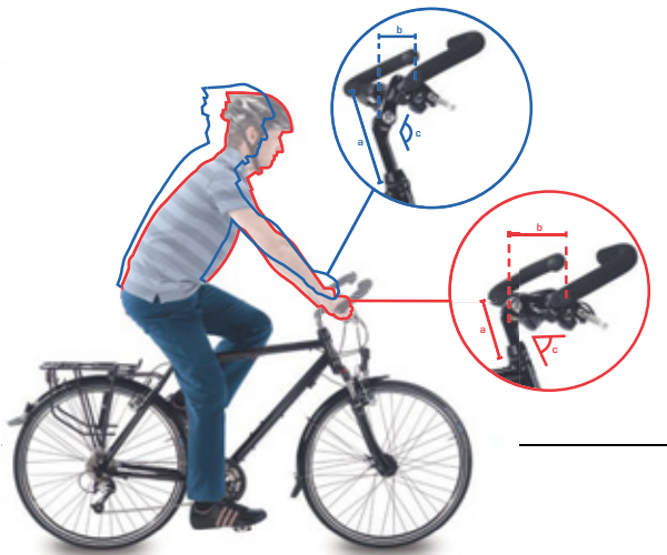
Figura 89: Posición de la bicicleta de ciudad (azul) y la bicicleta de trekking (rojo) mediante la modificación angular
