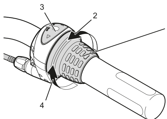
Figura 126: Ejemplo de uso del cambio de marchas SHIMANO Nexus
